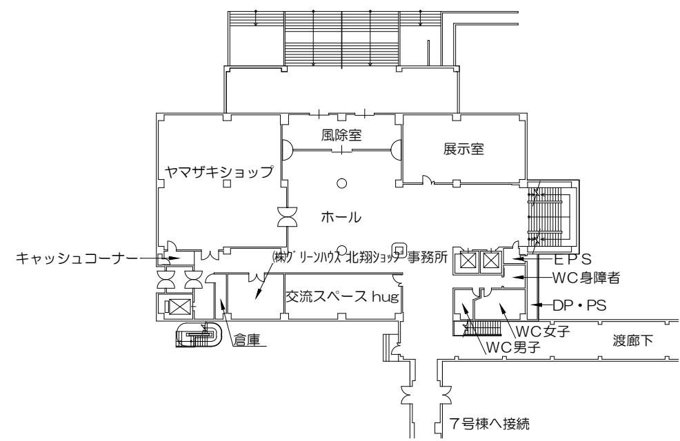
2階平面図
