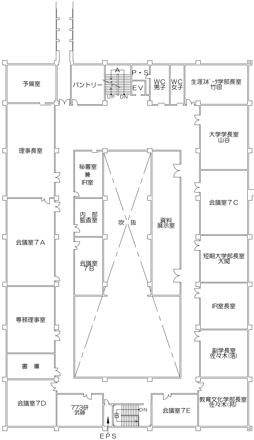
5階平面図
