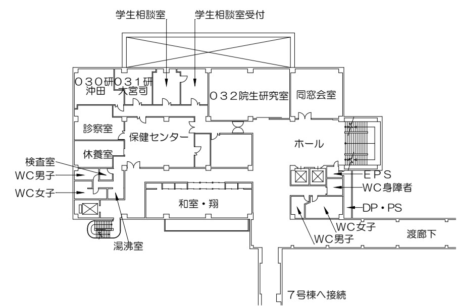
3階平面図
