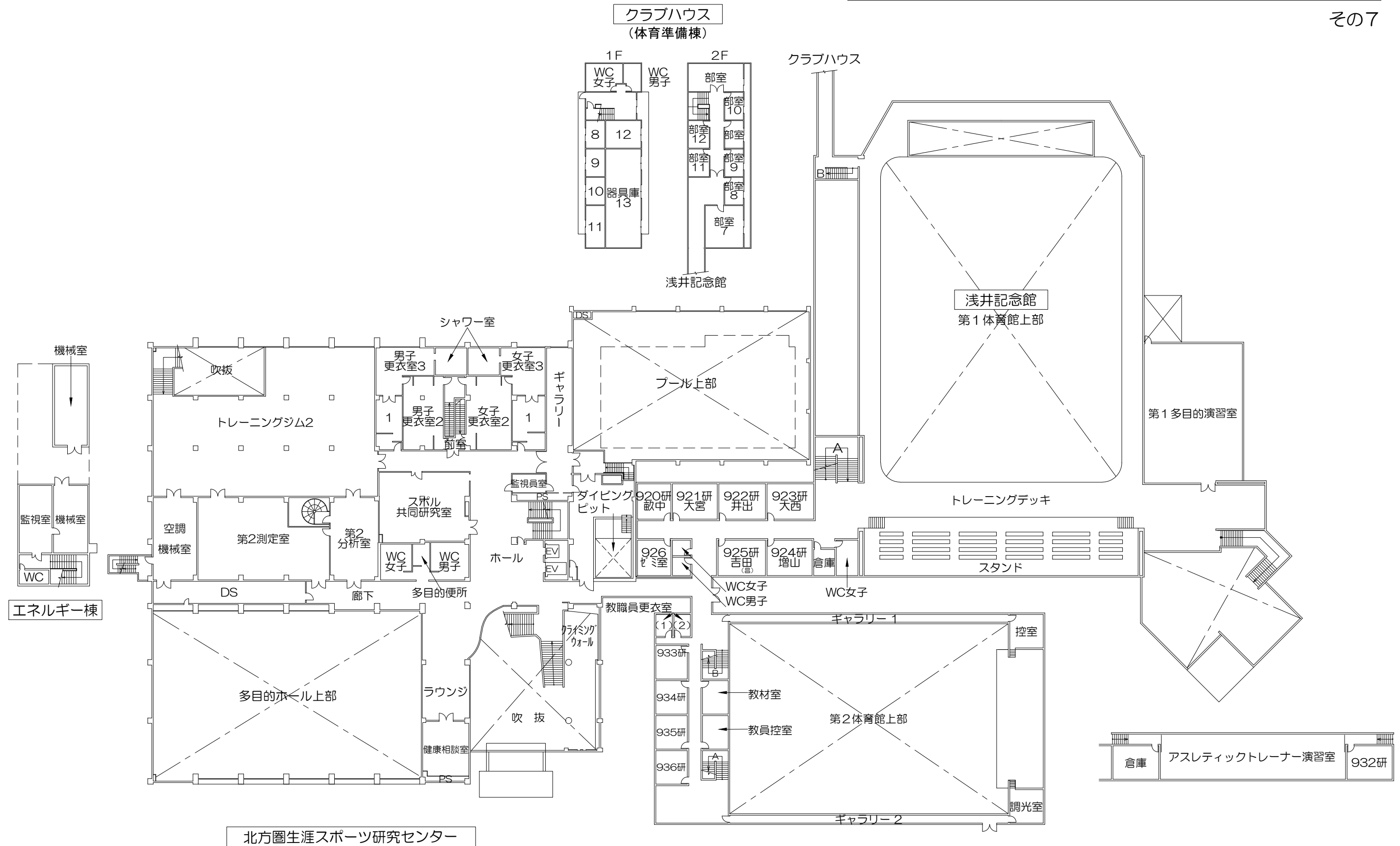
2階平面図
