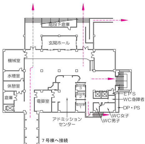
1 階平面図
