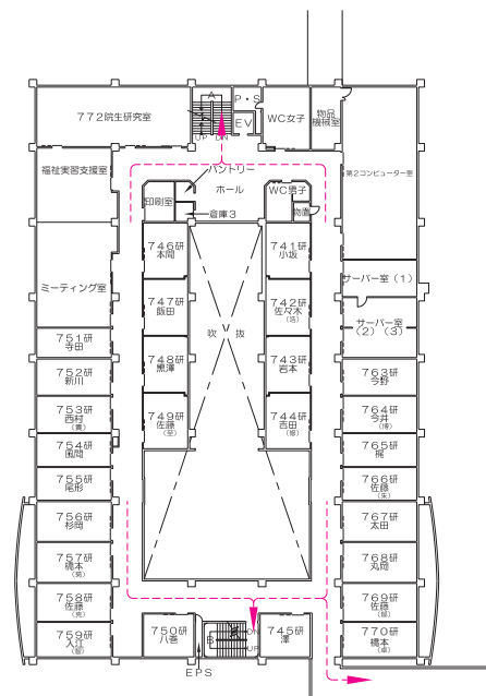
4 階平面図
