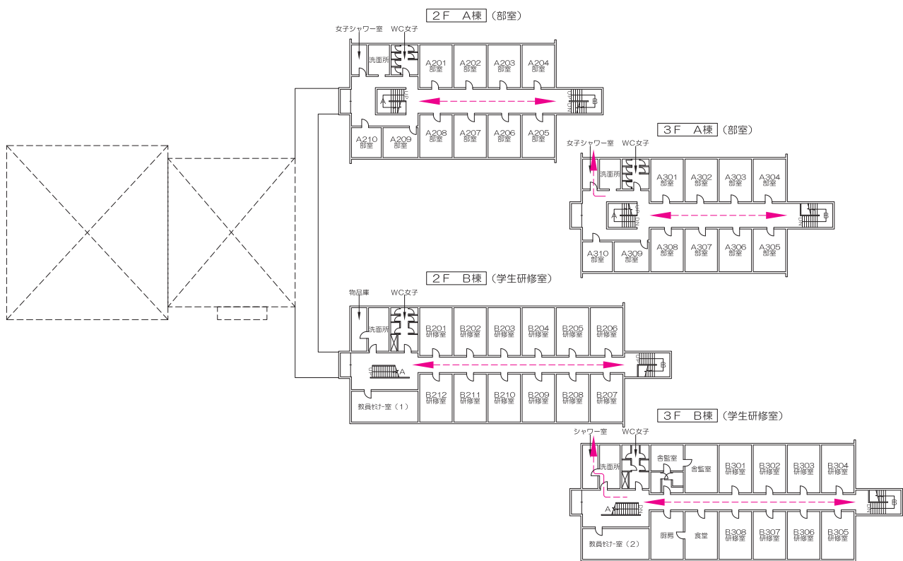
2・3 階平面図
