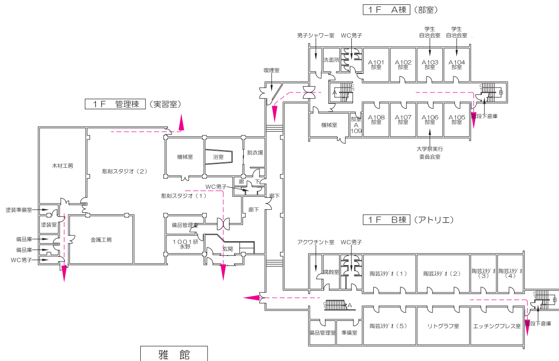
1 階平面図
