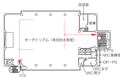
6 階平面図
