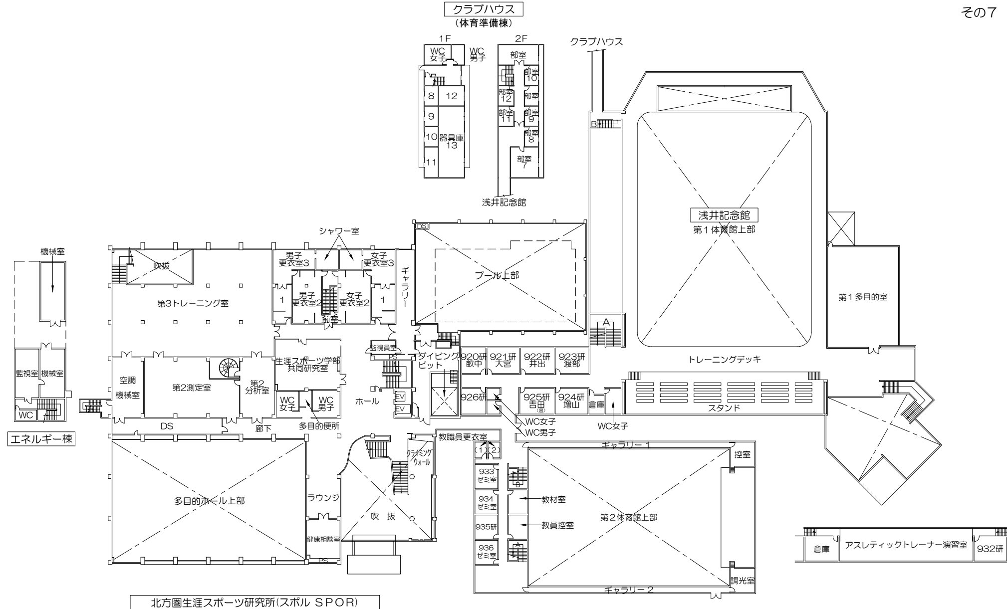
2階平面図
