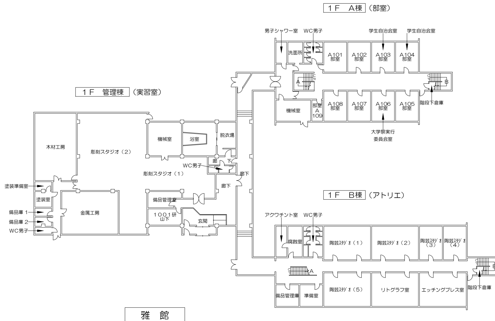
1 階平面図
