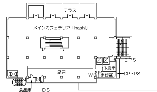
4階平面図
