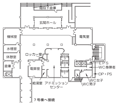
1階平面図
