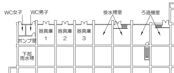
地下1階平面図
