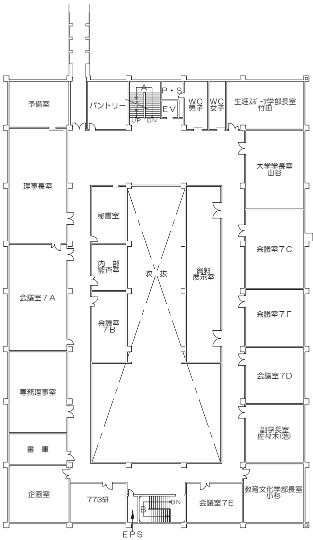
5階平面図
