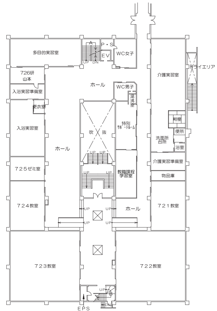
2階平面図
