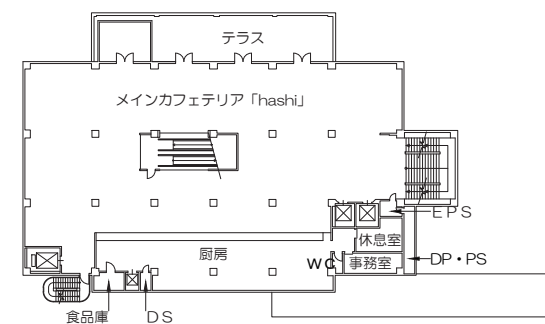
4階平面図
