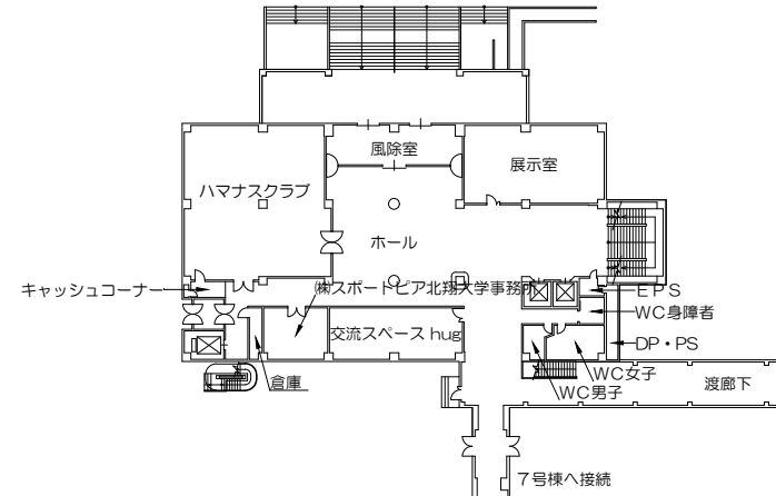
2階平面図
