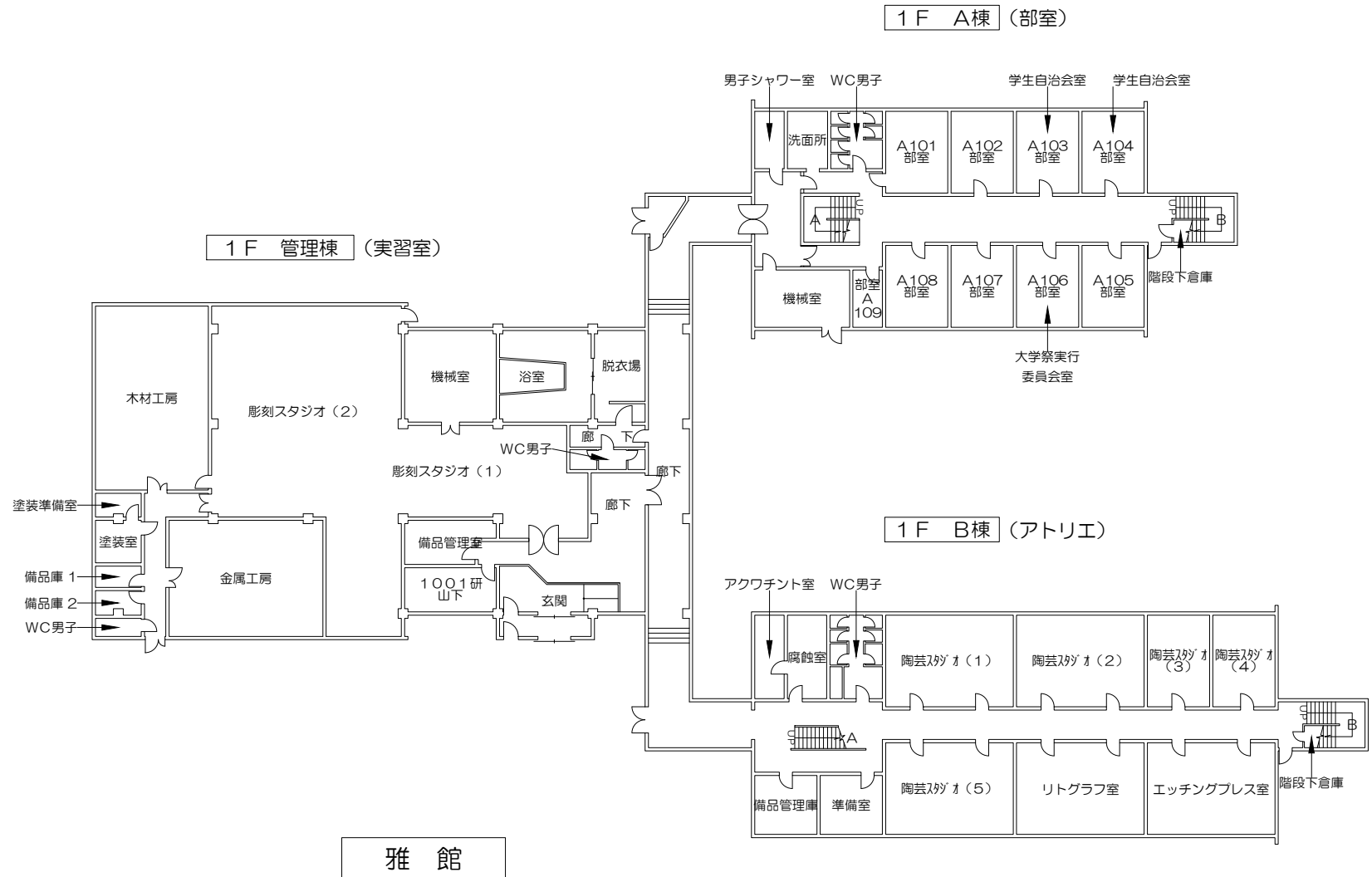
1階平面図
