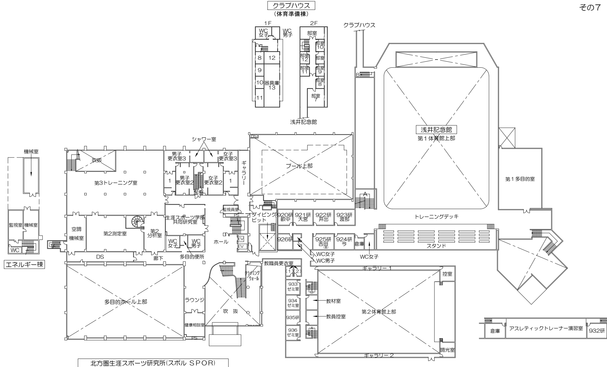
2階平面図
