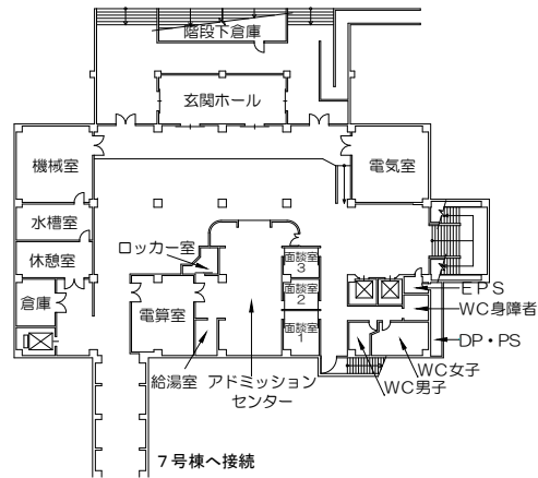
1階平面図
