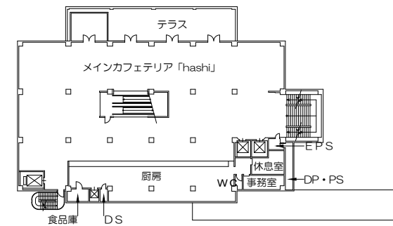
4階平面図
