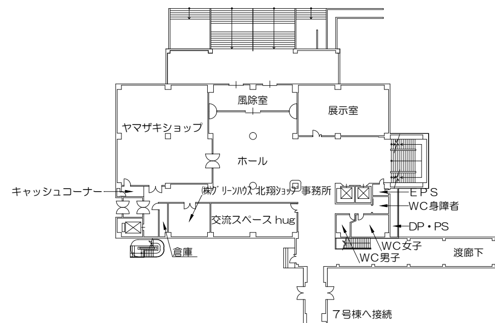
2階平面図
