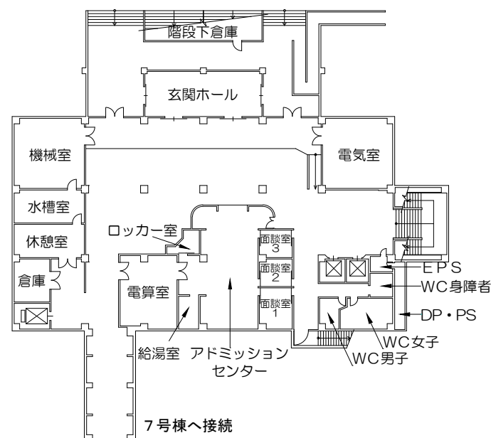
1階平面図
