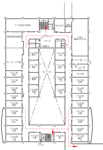
5階平面図
