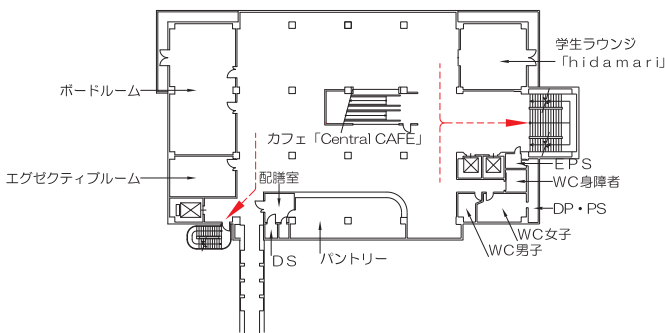
5 階
