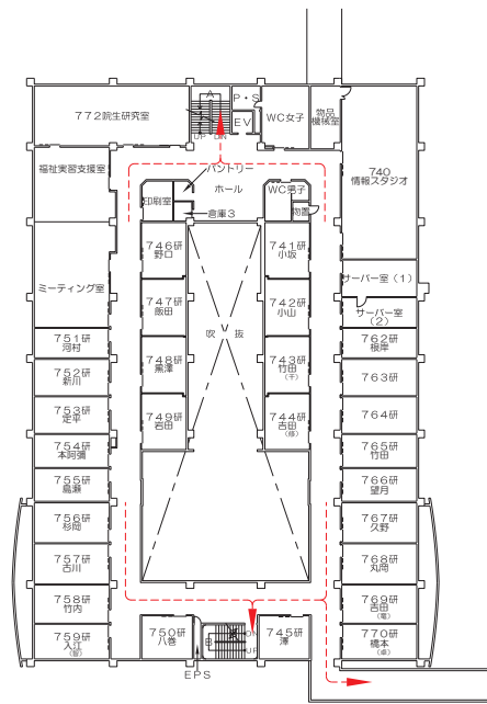
4階
