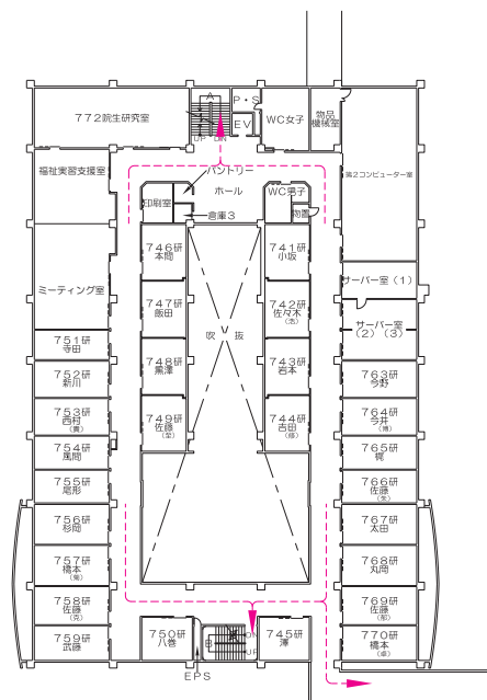
4 階平面図
