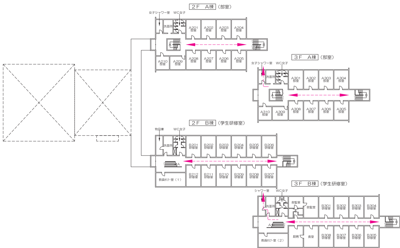
2・3 階平面図
