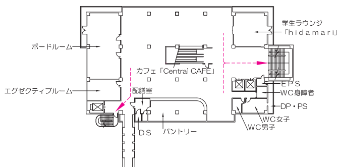
5 階平面図
