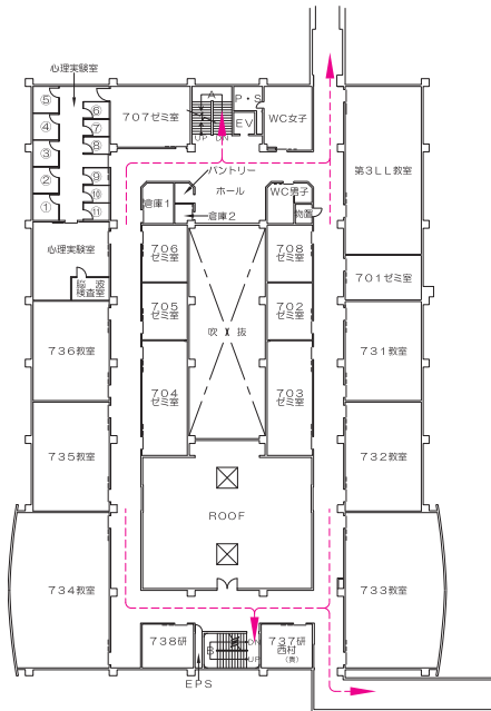
2階平面図
