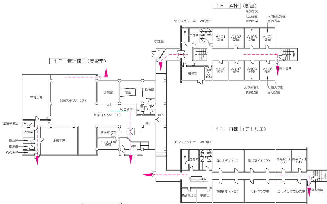
1 階平面図
