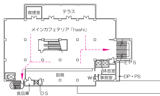
4 階平面図
