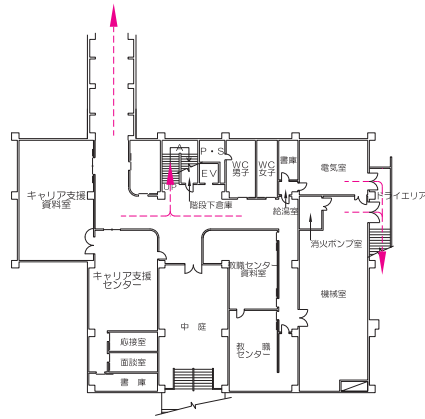
1階平面図
