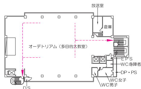
6 階平面図
