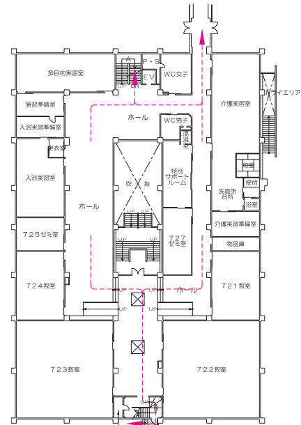
4階平面図
