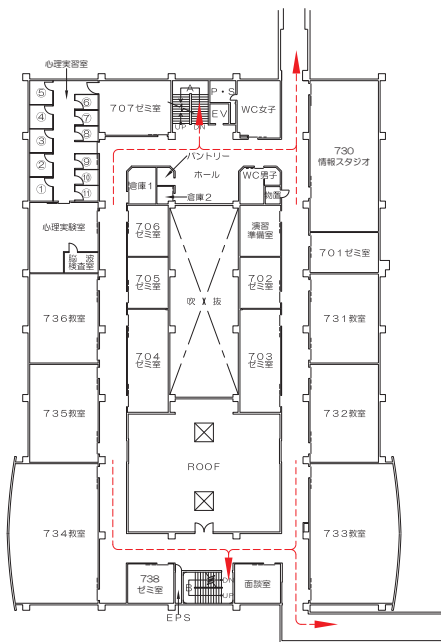
3 階平面図
