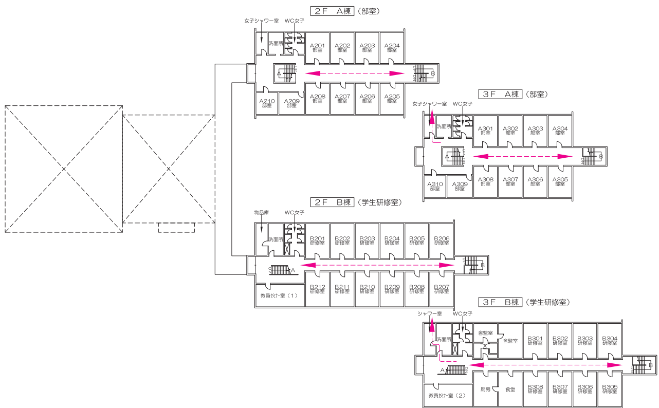
2・3 階平面図
