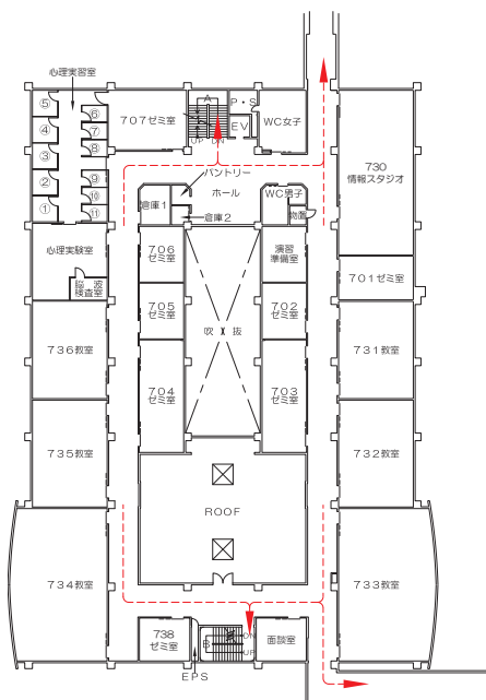
3階平面図
