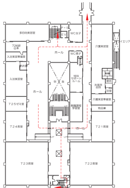
2階平面図
